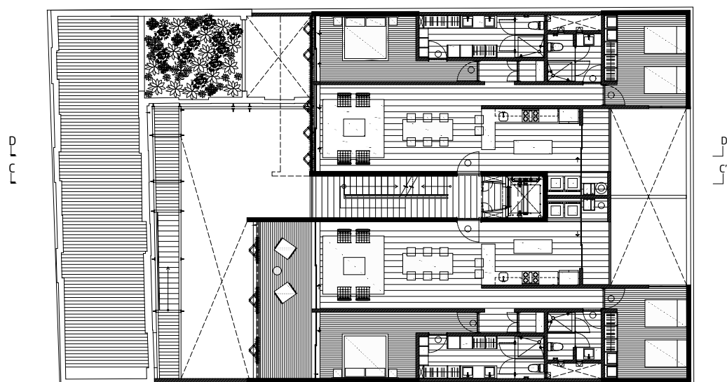
PLANTA 1º NIVEL
