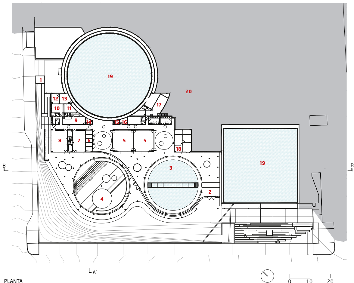
PLANTA
