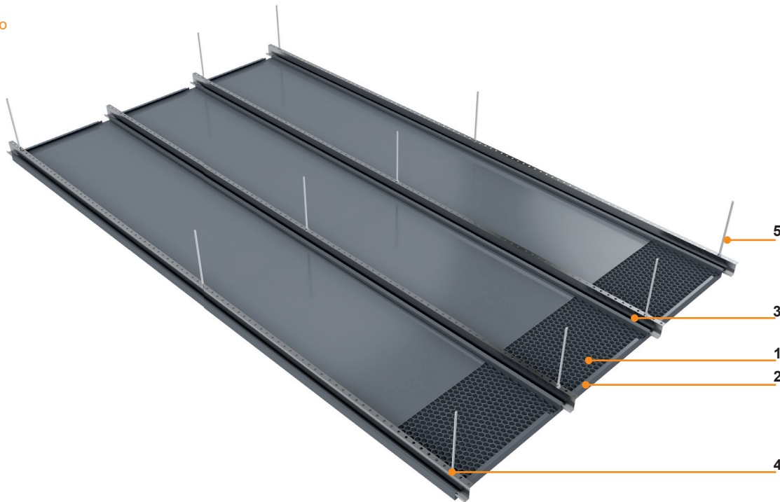
Isométrico
